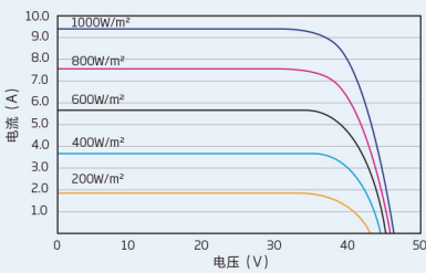
组件的I-V曲线(335W)
