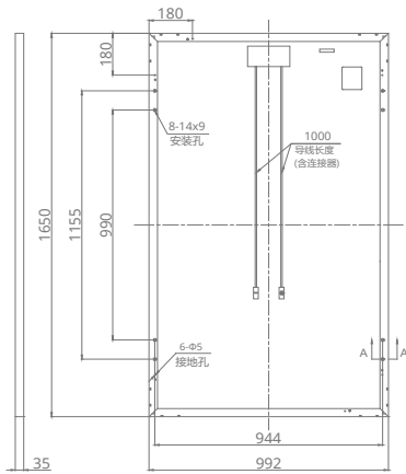
背面图
