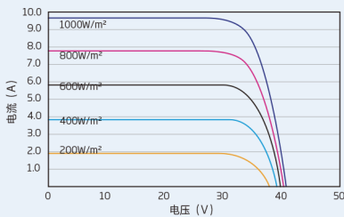
组件的I-V曲线 (305W)
